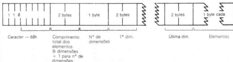
Figura C-8. Estrutura de uma matriz de caracteres
