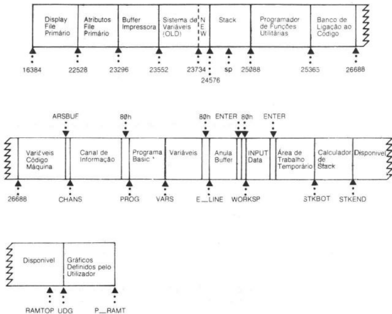
Figura C-1 — Estrutura de memória
