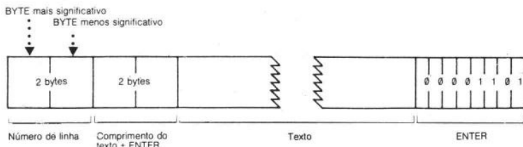
Figura C-2 — Estrutura da linha BASIC
