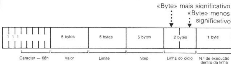
Figura C-6. Estrutura de um ciclo FOR/NEXT
