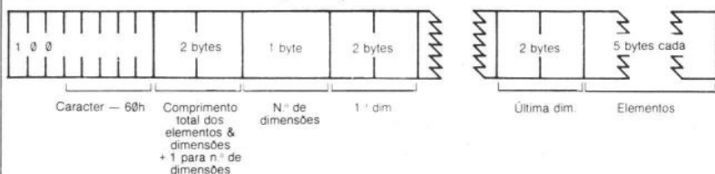
Figura C-5. Estrutura duma matriz numérica
