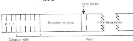
Figura C-3 — Número cujo nome é só uma letra
